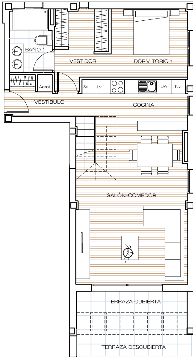
PLANTA BAJA
